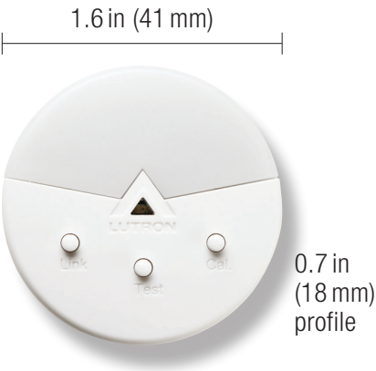
Shown actual size: Radio Powr Savr wireless daylight sensor in White (WH).
