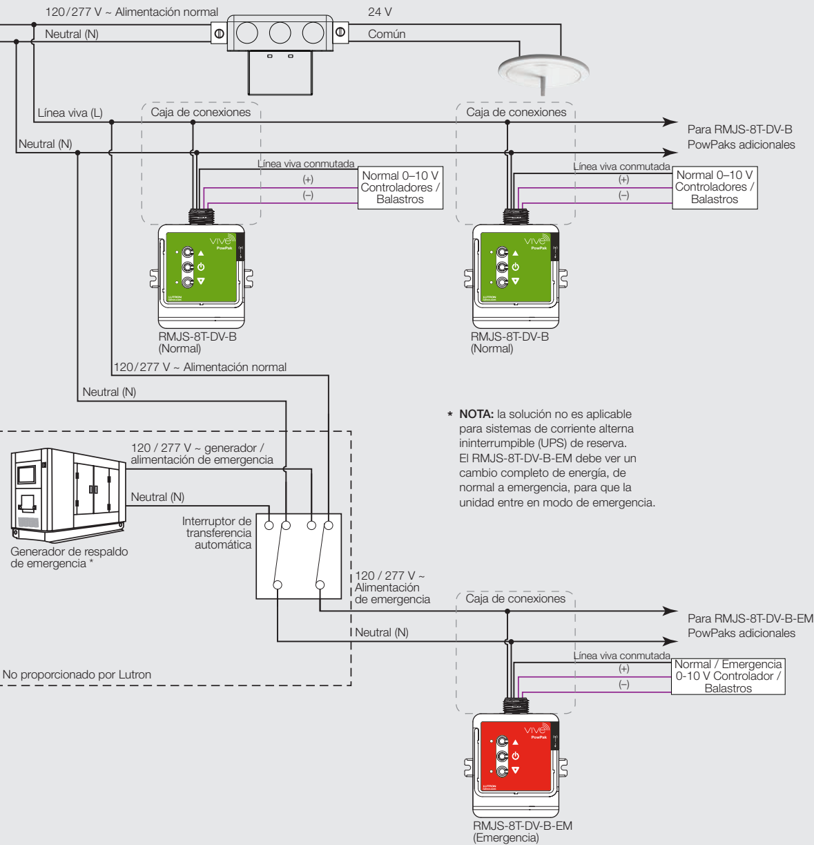
Diagrama de cableado del sistema (Hub Vive con PowPak de emergencia)
