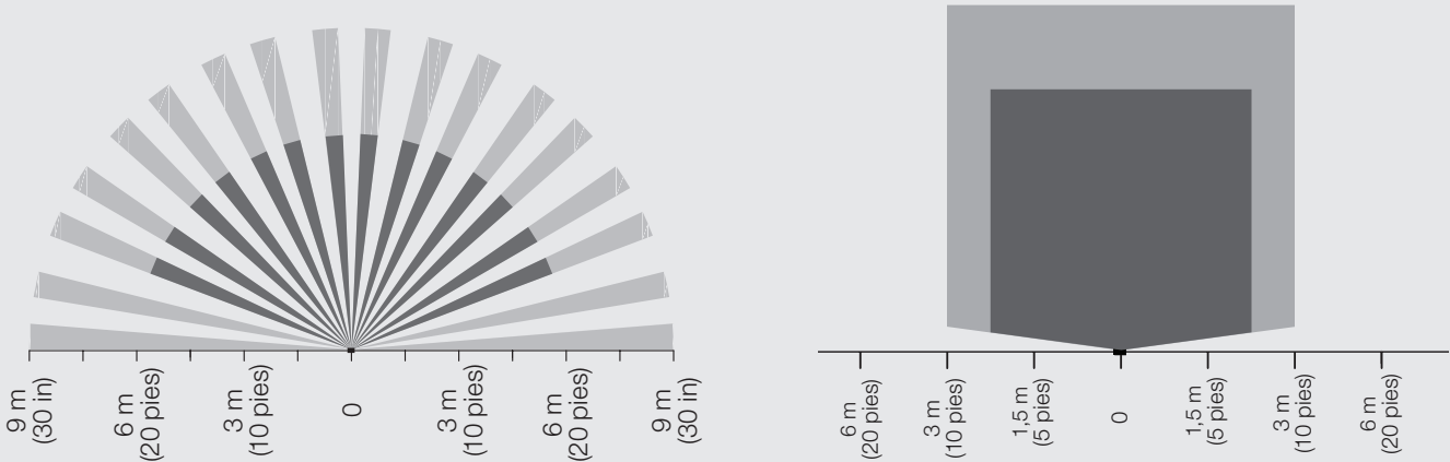
Diagrama del haz de PIR (solamente a modo de referencia)
