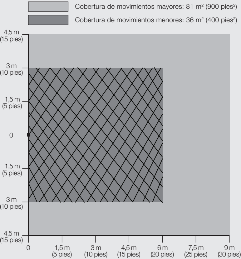
Cobertura de la rejilla de prueba NEMA WD7 (Ajuste de alta sensibilidad)
